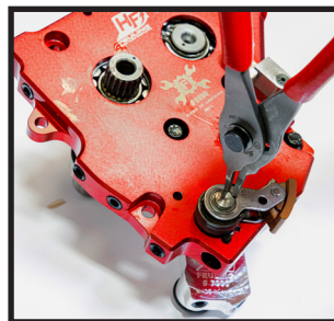
TENSIONER UNLOADER TOOL
